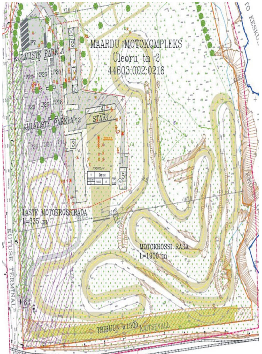
Üleoru tn 2 ning lähiala detailplaneeringu põhijoonis
